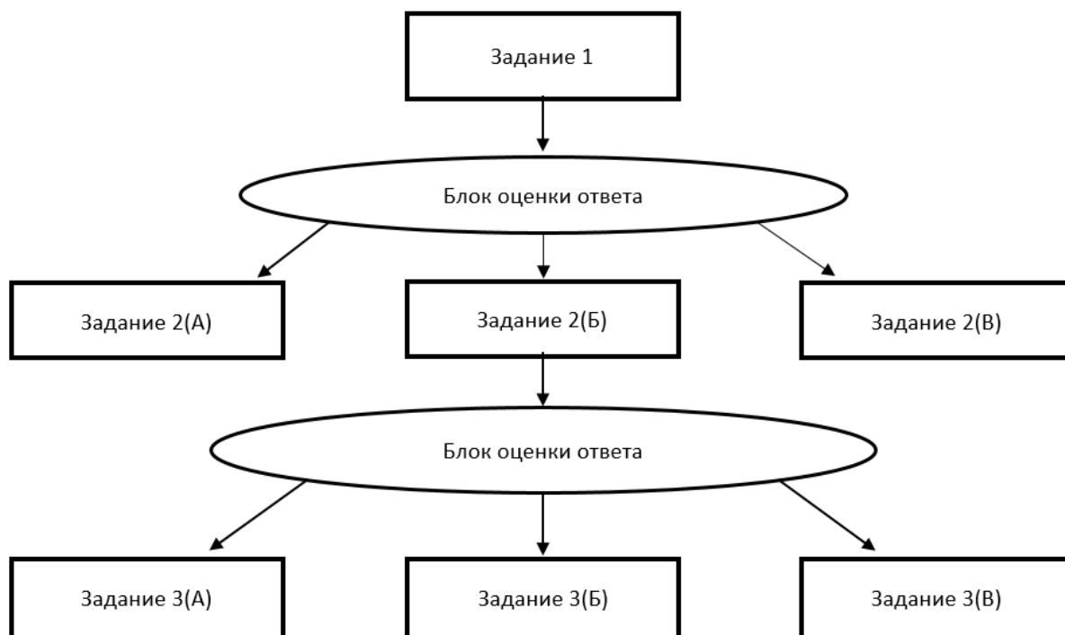
Рис2. Алгоритм отбора и предъявлений заданий (Многошаговая стратегия) (А- первый уровень сложности, Б – второй уровень сложности, В – третий уровень сложности)
